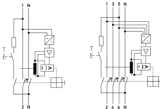
▲ zweipolig
